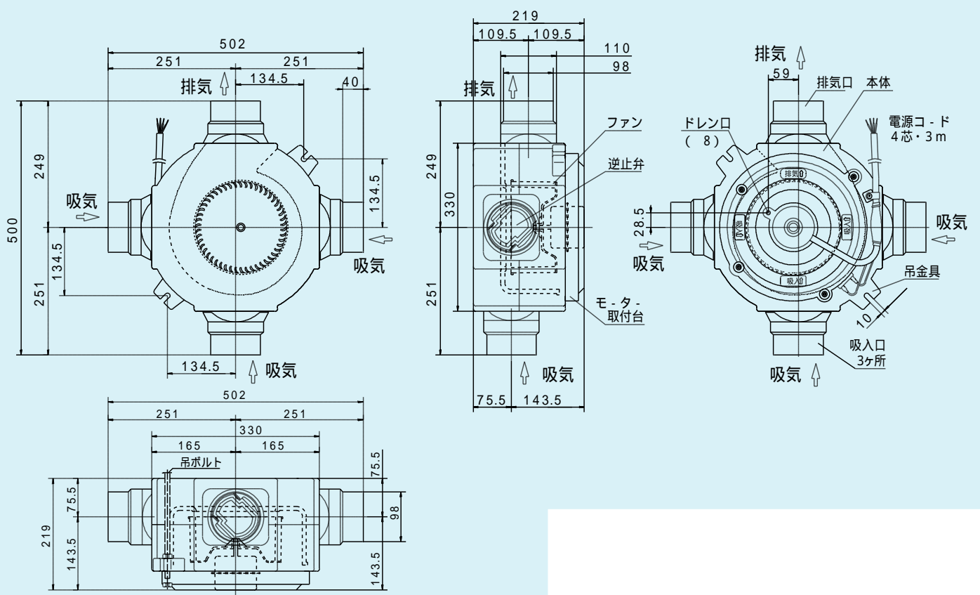
外形寸法図 < TSK-3R > (単位 : mm)
