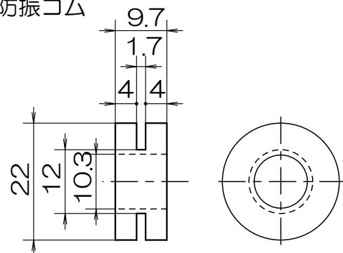
防振ゴム
