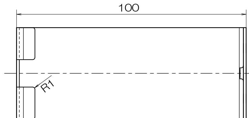
金具本体
