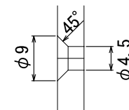
C穴詳細
