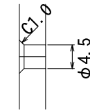
A穴詳細
