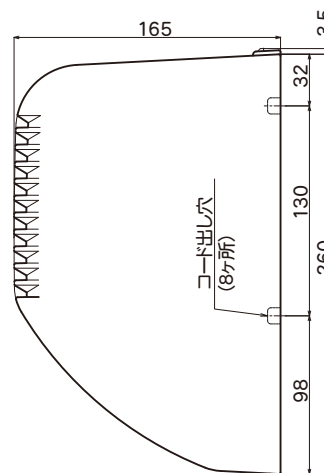
取付け穴寸法
