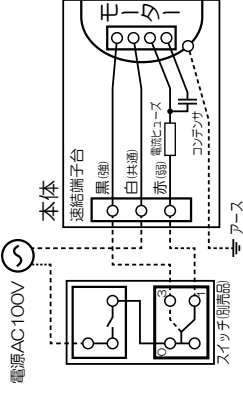
【配線図】
