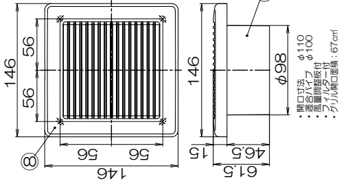
■副吸込口グリル(2個付属)
