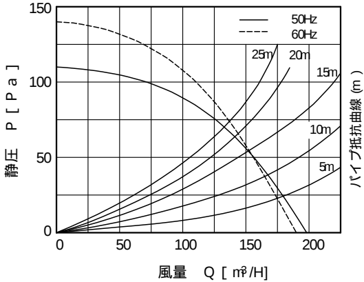
静圧・風量特性曲線
