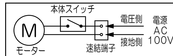
■結線図
