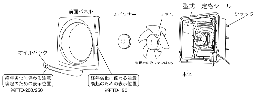
15cmオイルバック換気扇 FTD-150 (4枚羽根)
