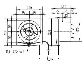
15cmオイルバック換気扇 FTD-150 (4枚羽根)
