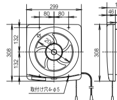
20cmオイルバック換気扇 FTD-200 (5枚羽根)
