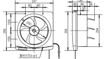
25cmオイルバック換気扇 FTD-250 (5枚羽根) FTD-250ES (5枚羽根)
