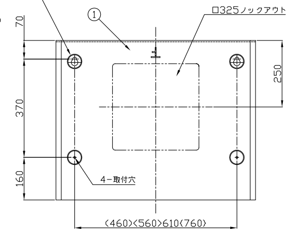
背面取付図
