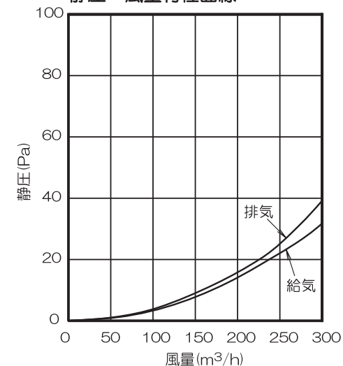
静圧・風量特性曲線
