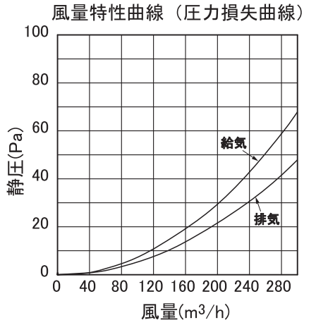
塩ビ管φ150×750mm装着時の風量試験
