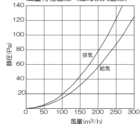
風量特性曲線 (圧力損失曲線)
