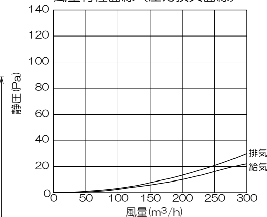
風量特性曲線 (圧力損失曲線)
