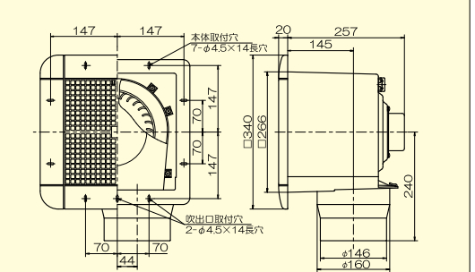
■ 本体寸法図 (単位: mm)
