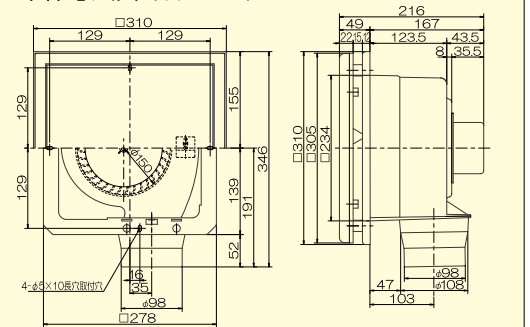
■ 本体寸法図 (単位: mm)
