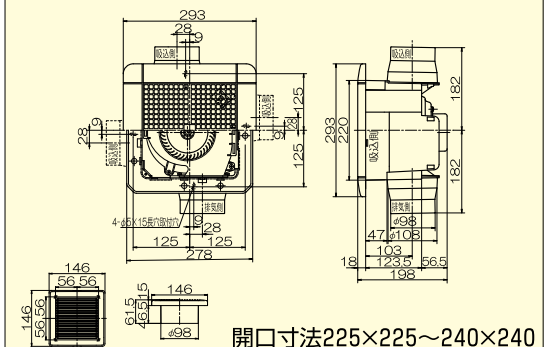
■ 本体寸法図 (単位: mm)
