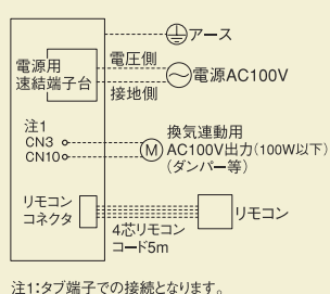
■配線例〈BF-231SHA〉
