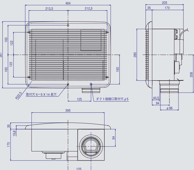
■外形寸法図〈BF-211SR〉(単位: mm)
