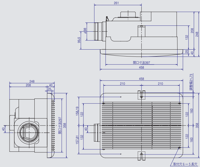
■外形寸法図〈BF-511SR〉(単位: mm)
