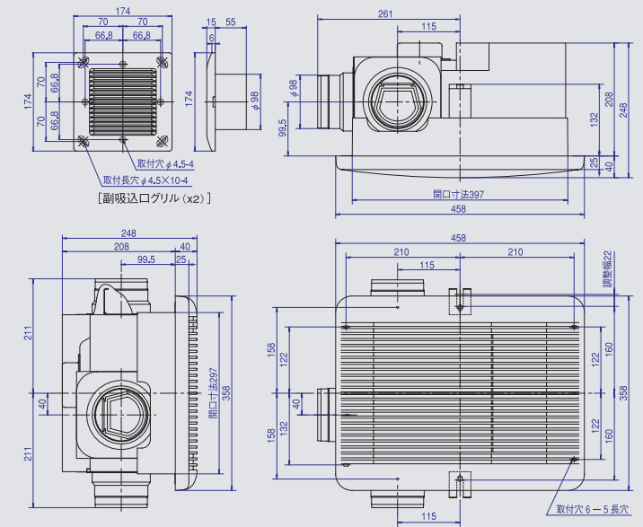
■外形寸法図〈BF-513SR〉(単位: mm)
