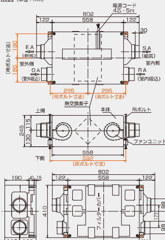
■外形寸法図 (単位: mm)
