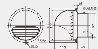
■外形寸法図 (単位: mm)
