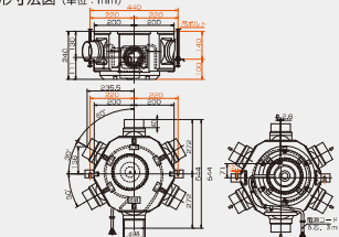
■外形寸法図 (単位: mm)
