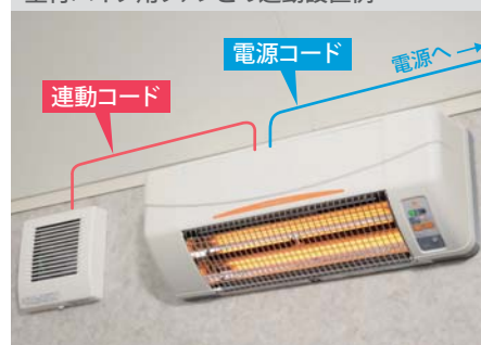
壁付パイプ用ファンとの連動設置例
