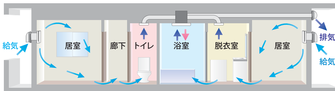
集合住宅(3室換気の場合)の24時間換気の空気の流れのイメージ図(BF-563RGD)
