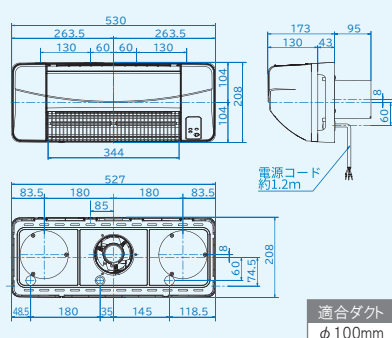
〈BF-961RGA〉(単位:mm)
