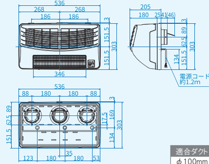
〈BF-871RGA2〉(単位:mm)
