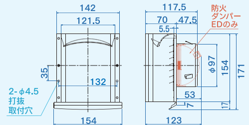
■外形寸法図(単位:mm)
