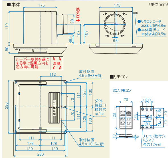
吹出口は奥側
