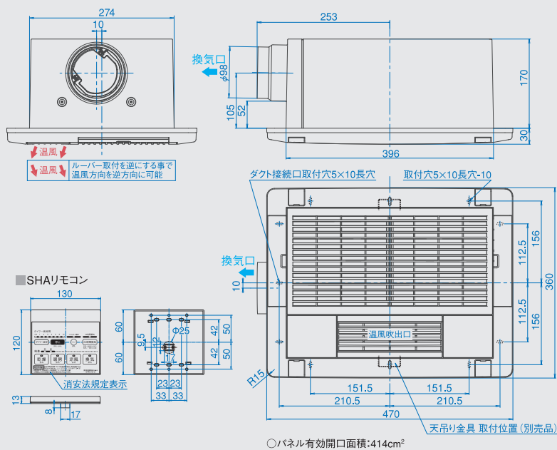
■外形寸法図〈BF-231SHA〉(単位:mm)
