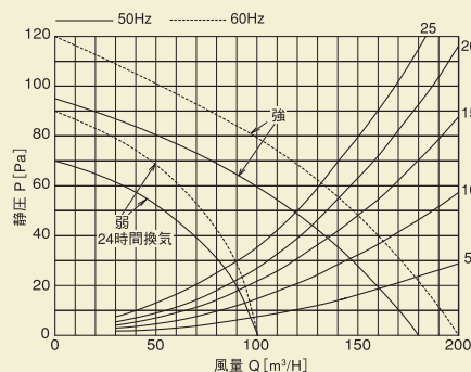
■静圧・風量特性曲線〈BF-231SHA〉
