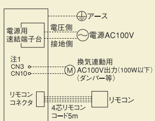
■配線例〈BF-231SHA〉
