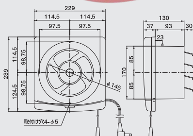
FTD-150 オイルパックタイプ
