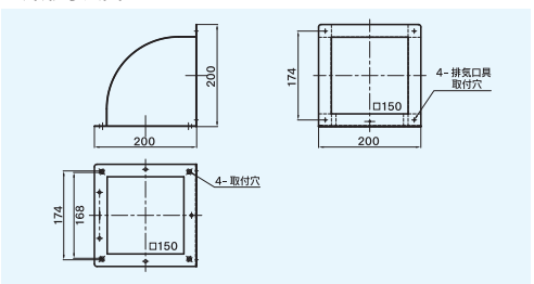
■外形寸法図 (単位：mm)
