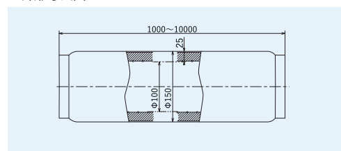
■外形寸法図 (単位: mm)
