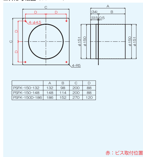
■外形寸法図 (単位: mm)
