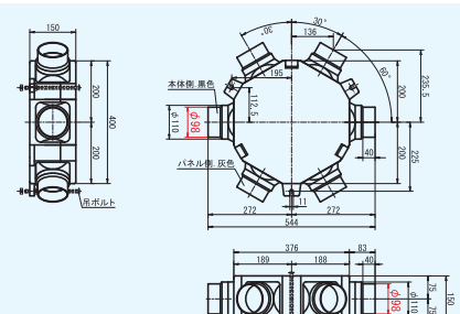
■外形寸法図 (単位: mm)
