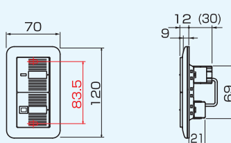
■外形寸法図 (単位: mm)
