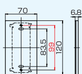
■外形寸法図 (単位: mm)
