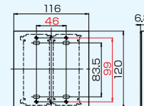
■外形寸法図 (単位: mm)
