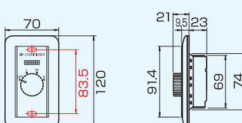
■外形寸法図 (単位: mm)
