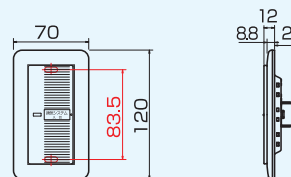
■外形寸法図 (単位: mm)
