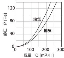
■圧力損失曲線
