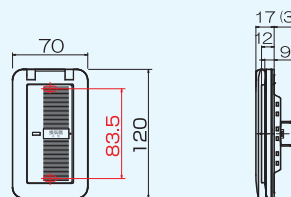
■外形寸法図 (単位: mm)
