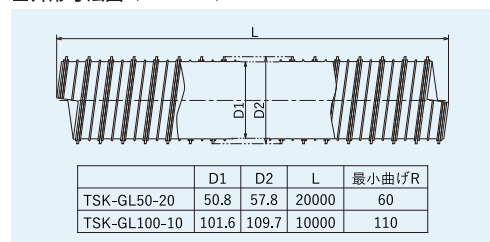
■外形寸法図 (単位: mm)
