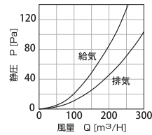
■圧力損失曲線
