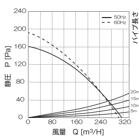
■静圧・風量特性曲線
