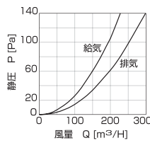
■圧力損失曲線
