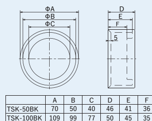
■外形寸法図 (単位: mm)
