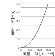
■圧力損失曲線
