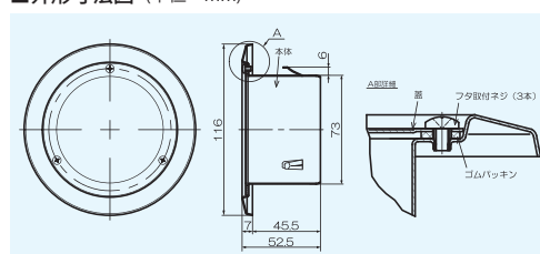
■外形寸法図 (単位: mm)
