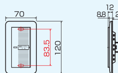
■外形寸法図 (単位: mm)
