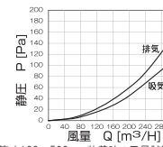
■圧力損失曲線
