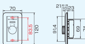
■外形寸法図 (単位: mm)
