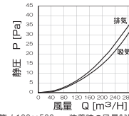
■圧力損失曲線
