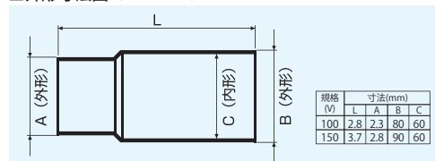
■外形寸法図 (単位: mm)
