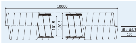
■外形寸法図 (単位: mm)
