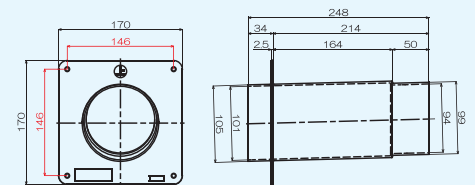
■外形寸法単位：mm
