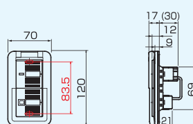
■外形寸法図 (単位: mm)
