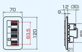
■外形寸法図 (単位: mm)
