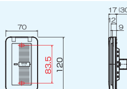
■外形寸法図 (単位: mm)
