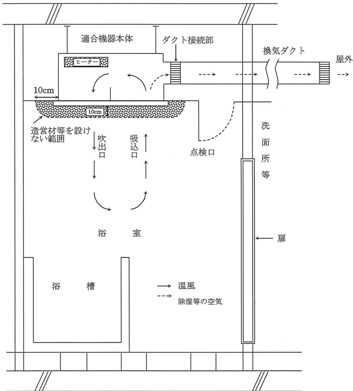
浴室に設ける天井組込み形衣類乾燥機・暖房等用電気機器の設置図
