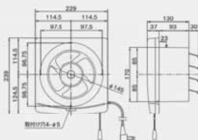
FTD-150 オイルバックタイプ
