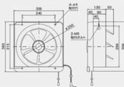
FTK-250/250ES 金属タイプ
